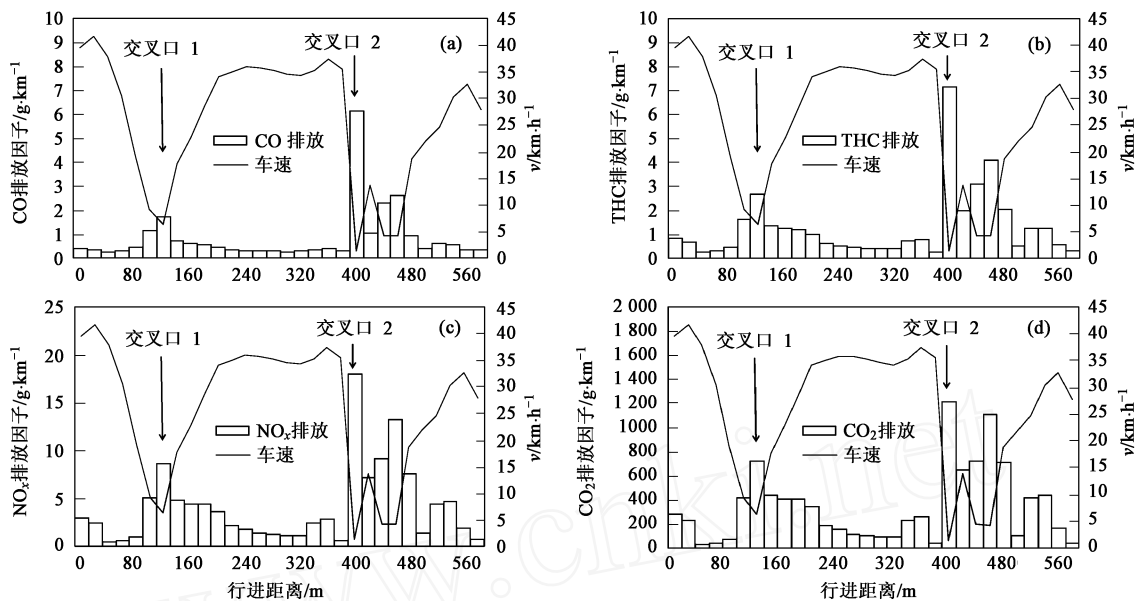
图 5 轻型柴油车在微观街道上的污染物排放水平随车速的变化
