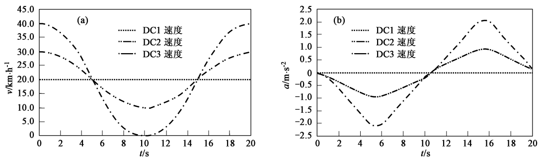
图 6 平均车速为 20 \text{ km} \cdot \text{h}^{-1} 时的 3 种驾驶方式的速度、加速度模拟曲线
