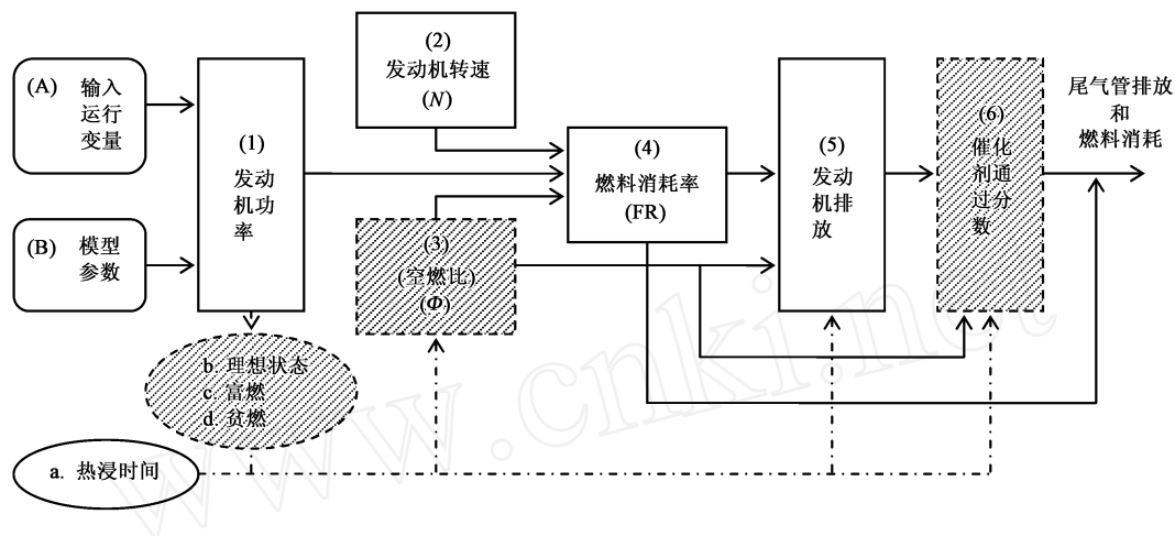
虚线框与阴影部分为汽油车专用模块
