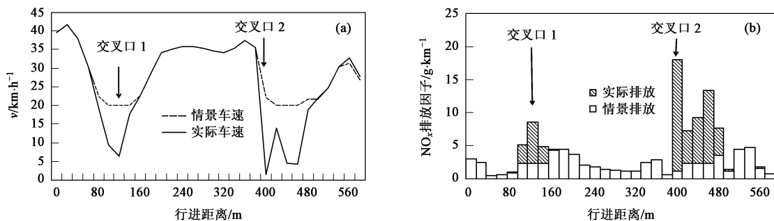
图10 交通改善情景下轻型柴油车车速以及 NO x 排放水平瞬时变化与实际情况的比较
