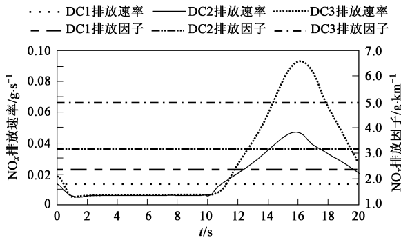
图7 3种驾驶方式下的 NO x 排放速率与排放因子的模拟结果比较
