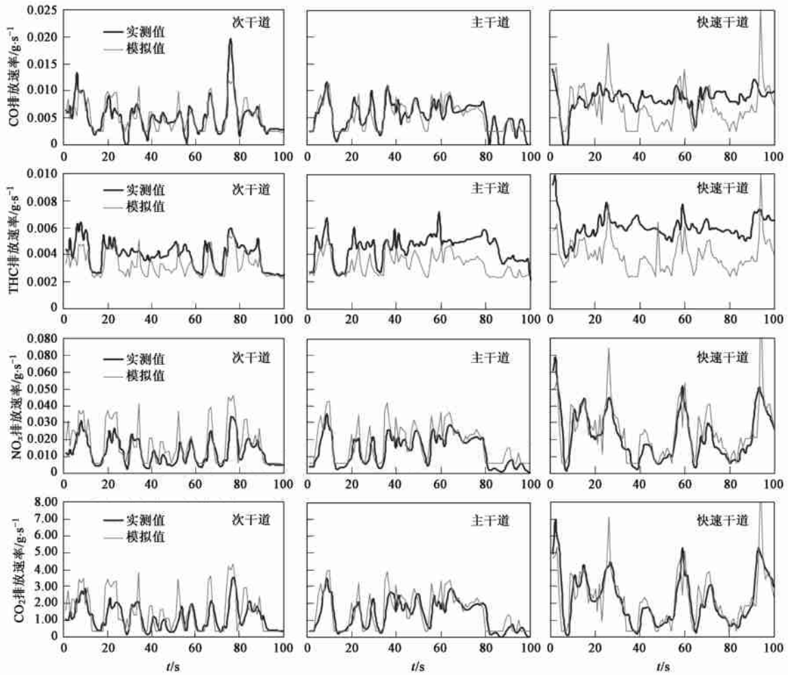
图3 测试车辆污染物瞬时排放速率实测结果与模拟值比较
