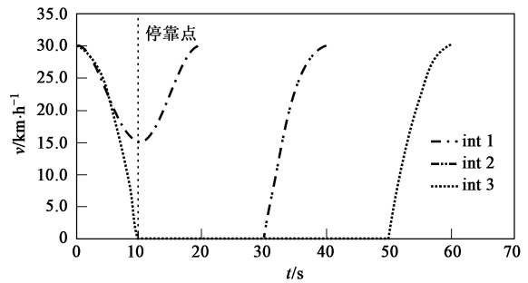
图8 车辆在3种信号灯等候时间条件下的车速模拟曲线
