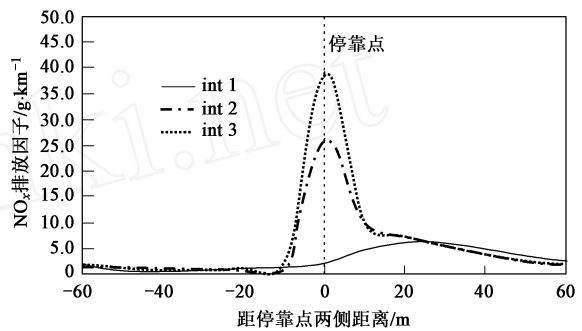
图9 车辆在3种信号灯等候时间条件下的 NO x 排放因子的模拟结果比较
